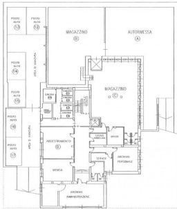
PIANTA PIANO INTERRATO Sc. 1:200
